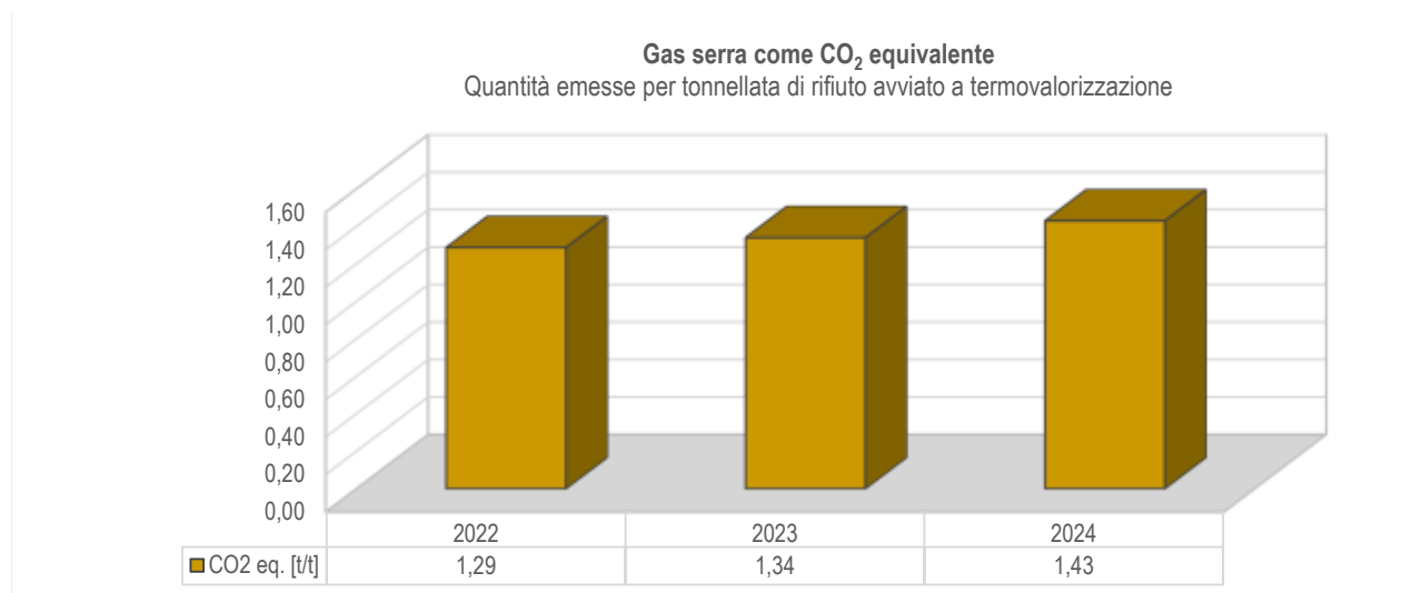
Figura 25: Emissione specifica di Gas Serra nell'ultimo triennio
