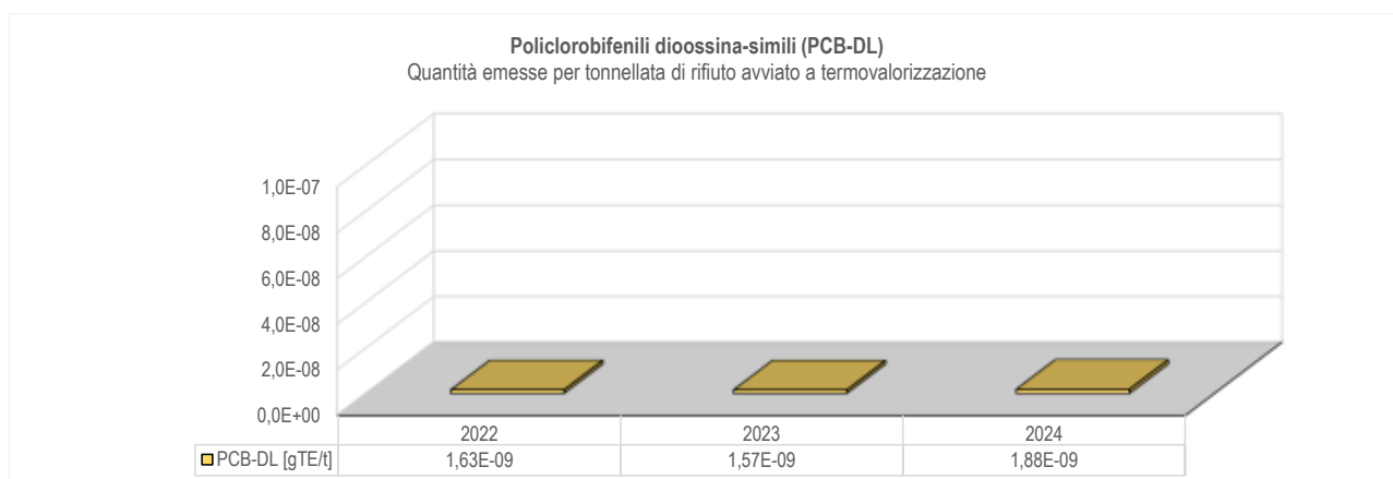
Figura 32: Emissione specifica di Policlorobifenili diossina-simili nell'ultimo triennio – monitoraggio mediante campionamento a lungo termine
