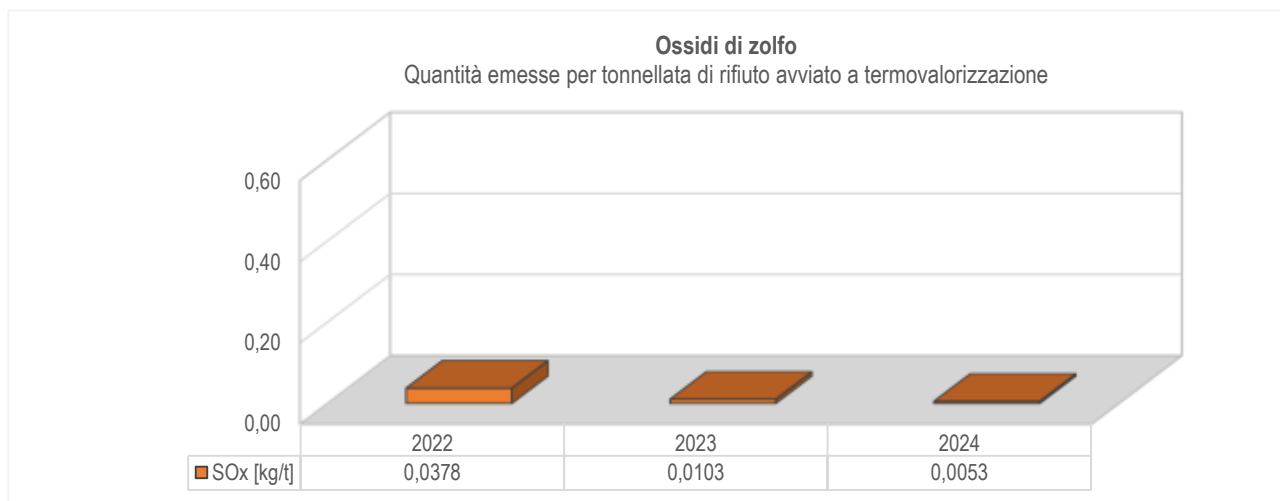
Figura 19: Emissione specifica di Ossidi di Zolfo nell'ultimo triennio
