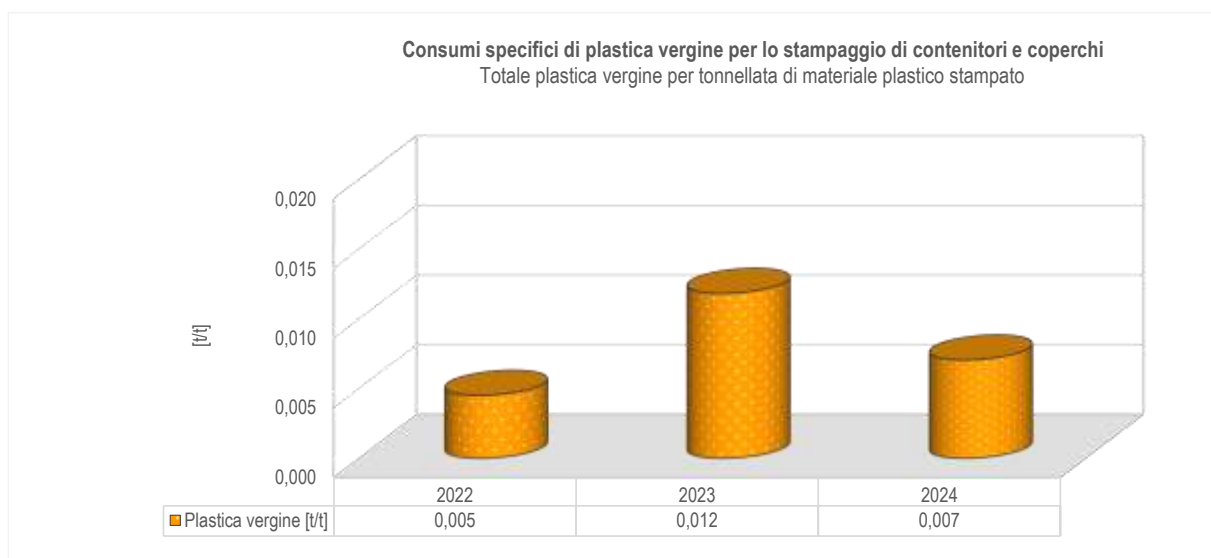
Figura 41: Consumi specifici di plastica vergine per lo stampaggio nell'ultimo triennio
