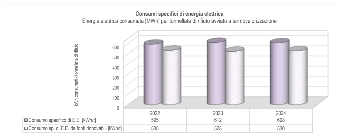
Figura 51: Consumo specifico di energia elettrica nell'ultimo triennio
