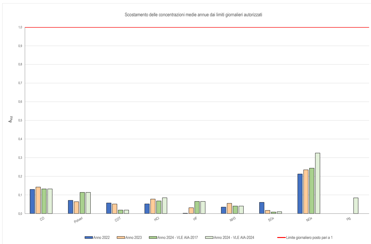
Figura 14: Andamento dello scostamento delle concentrazioni medie annue dal valore limite autorizzato nell'ultimo triennio
