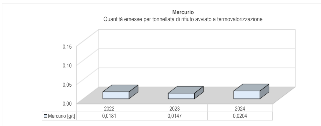
Figura 24: Emissione specifica di Mercurio nell'ultimo triennio
