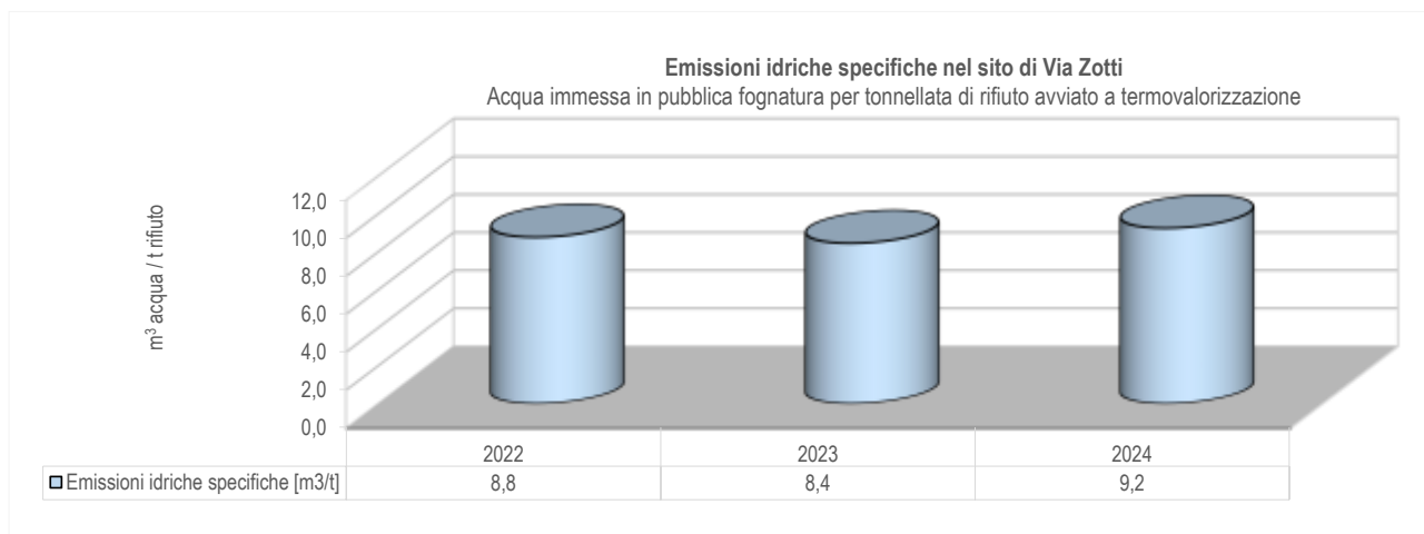
Figura 35: Emissioni idriche specifiche nell'ultimo triennio
