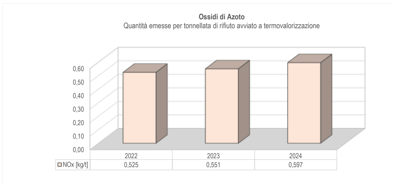
Figura 18: Emissione specifica di Ossidi di Azoto nell'ultimo triennio
