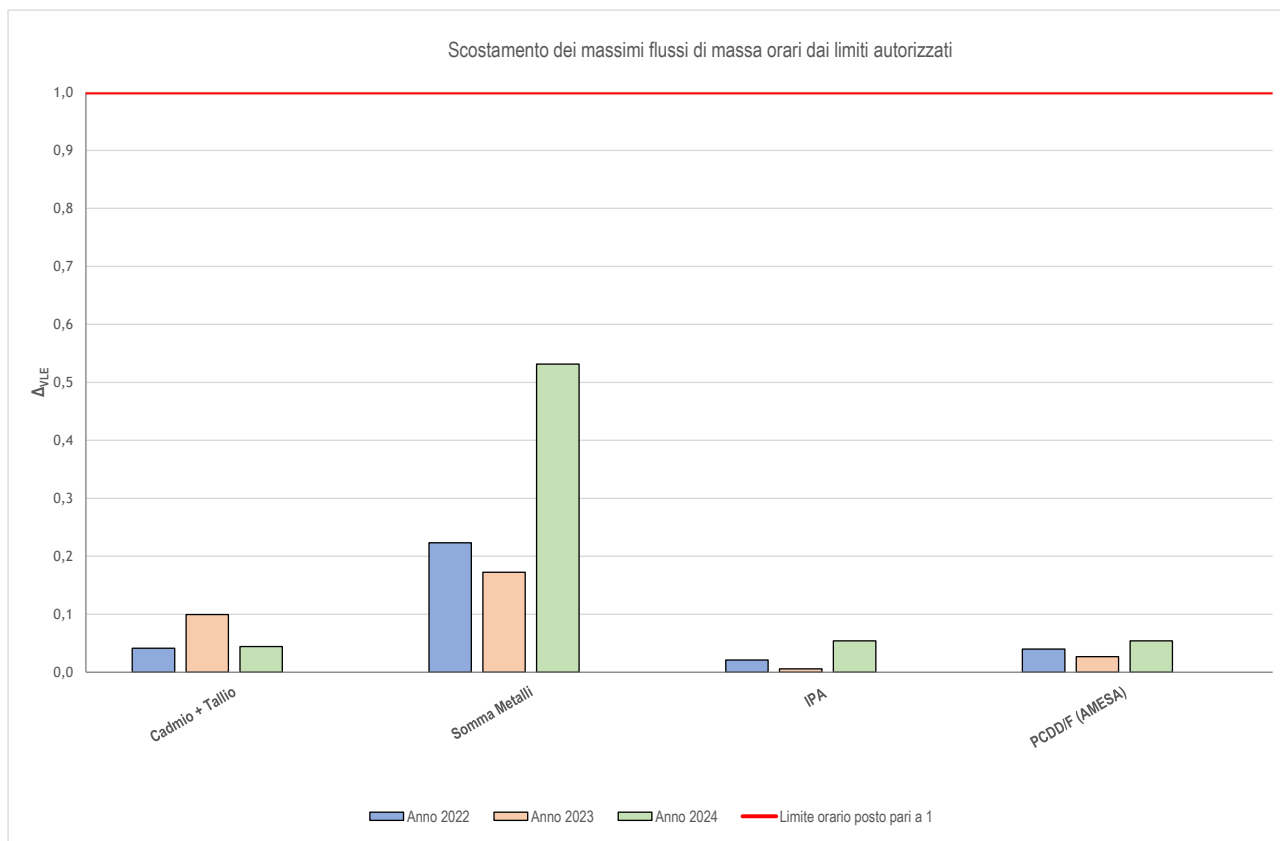
Figura 27: Andamento dello scostamento dei massimi flussi di massa dal valore limite autorizzato nell'ultimo triennio
