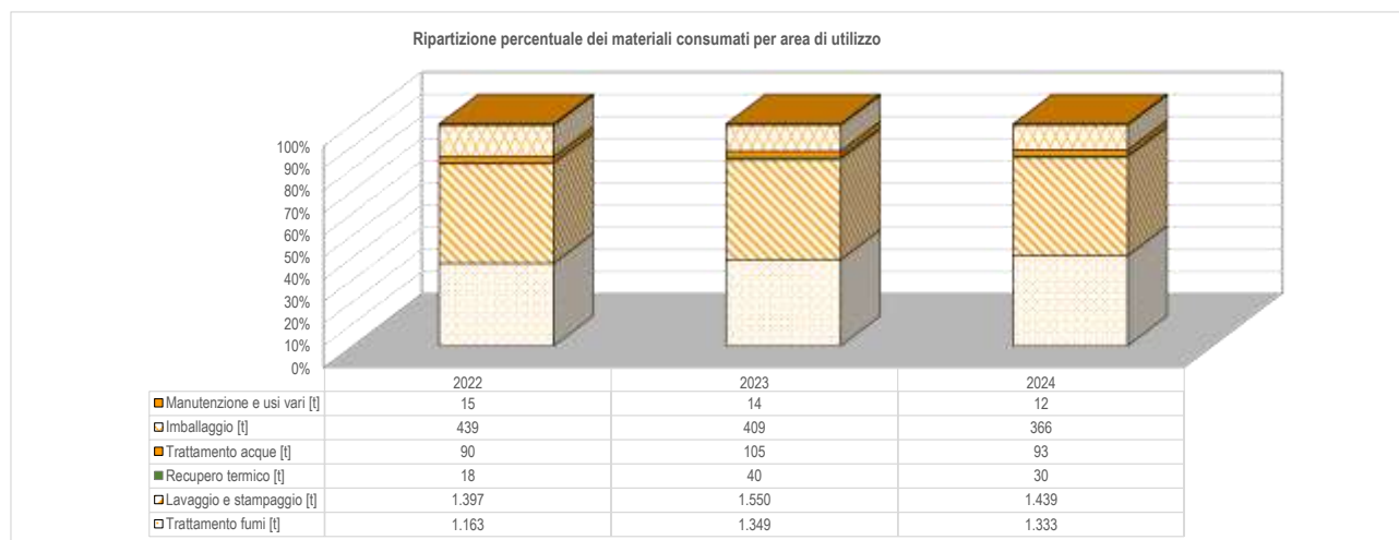
Figura 37: Ripartizione di materie prime, ausiliari e materiali nell'ultimo triennio
