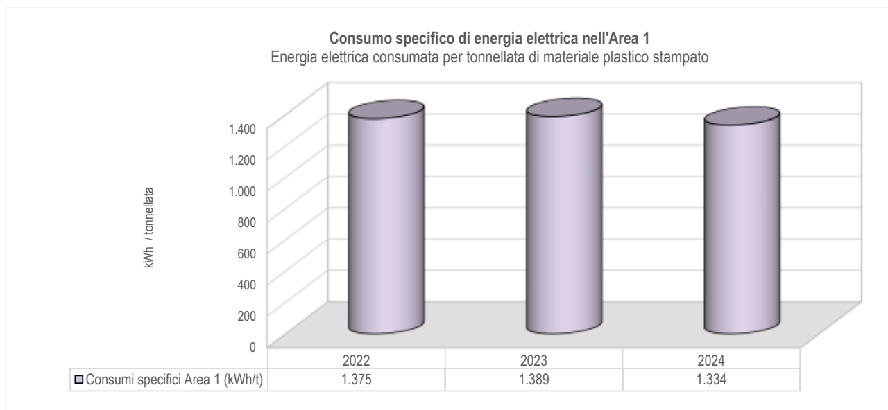
Figura 49: Consumo specifico di energia elettrica per la totalità dell'Area 1 nell'ultimo triennio
