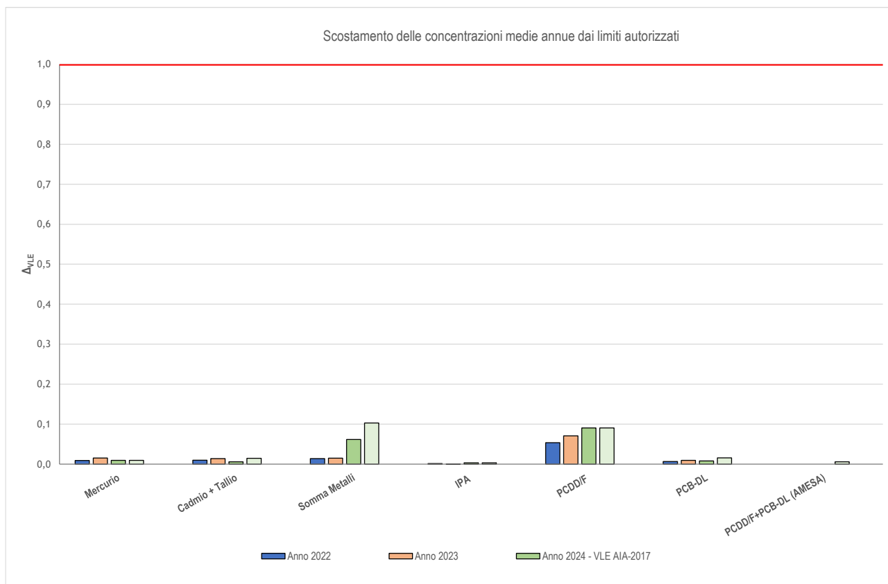
Figura 26: Andamento dello scostamento delle concentrazioni dal valore limite autorizzato nell'ultimo triennio
