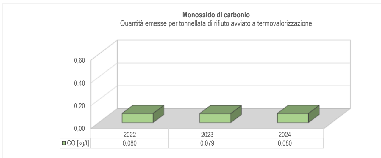
Figura 17: Emissione specifica di Monossido di carbonio nell'ultimo triennio
