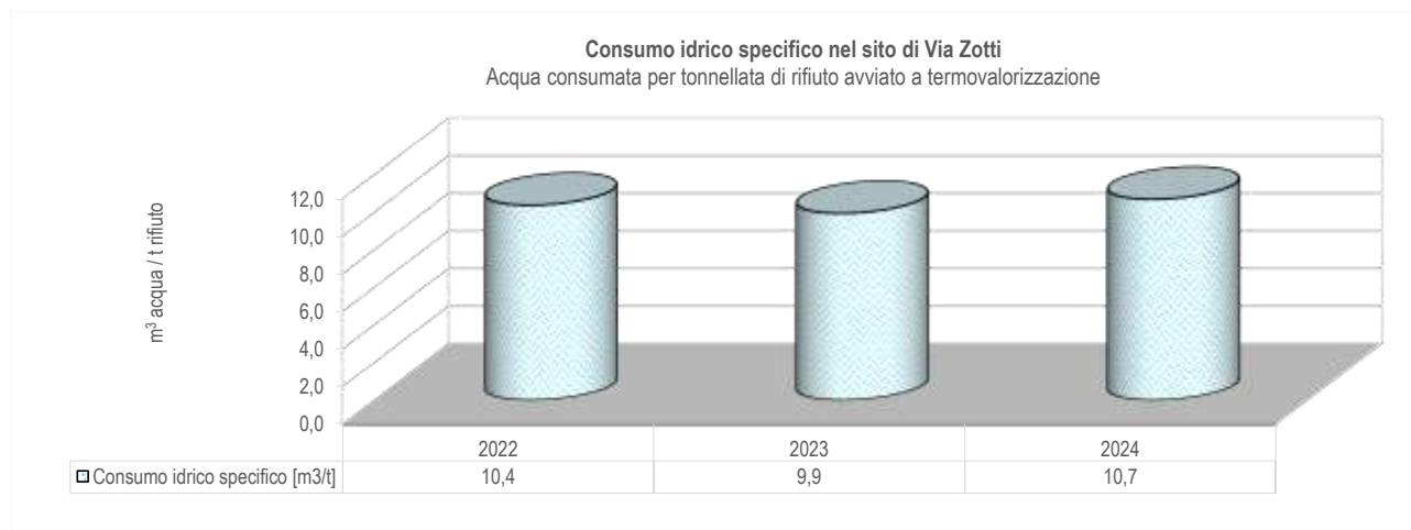
Figura 34: Consumo idrico specifico nell'ultimo triennio
